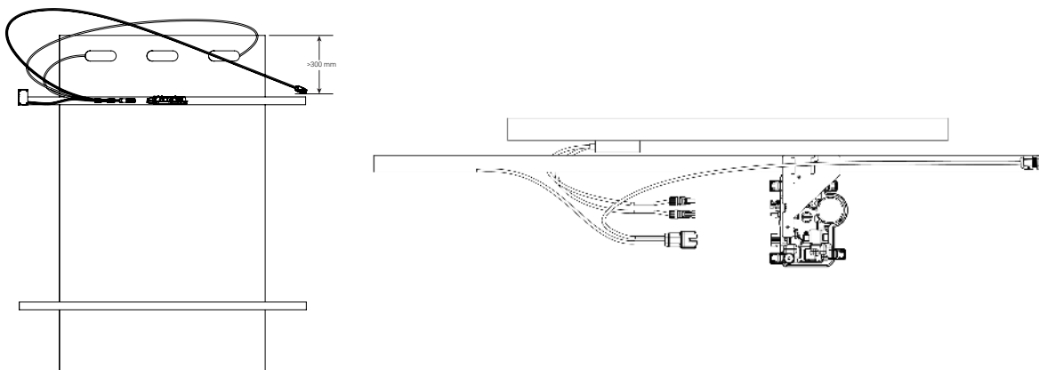
Illustration 3 : Montage vertical
